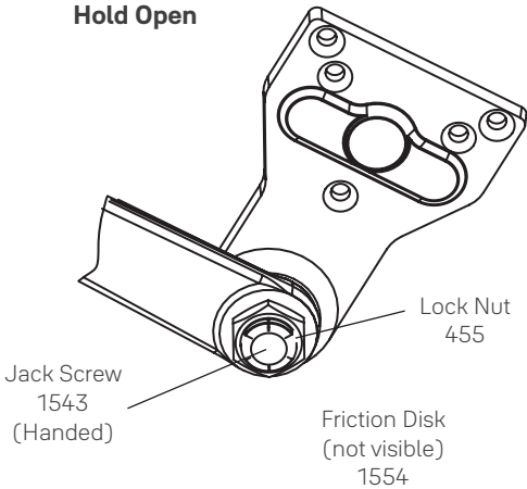
Hold Open
